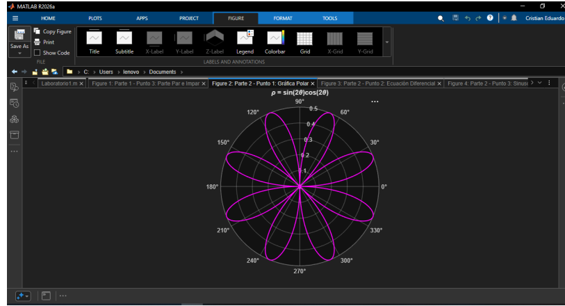
Figura 10: Gráfica polar de \rho = \sin(2\theta) \cos(2\theta) .
