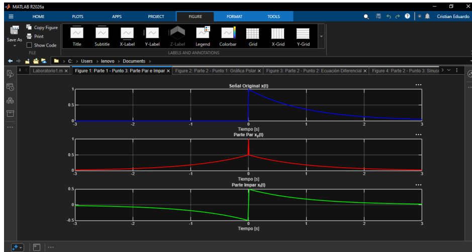
Figura 9: Descomposición en parte par e impar de la señal x(t) = e^{-t}u(t) .
